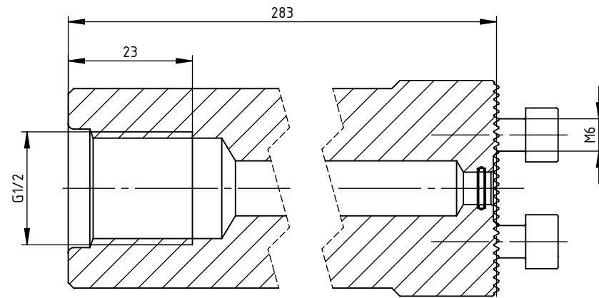
SCHNITT B-B
