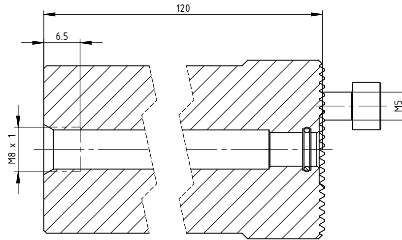
SCHNITT A-A
