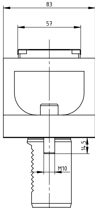
ANSICHT A
