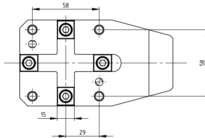
ANSICHT A
