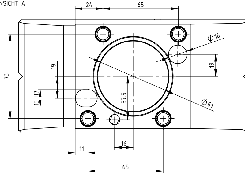
ANSICHT A
