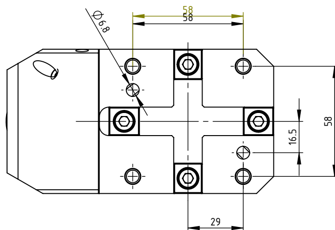
ANSICHT A
