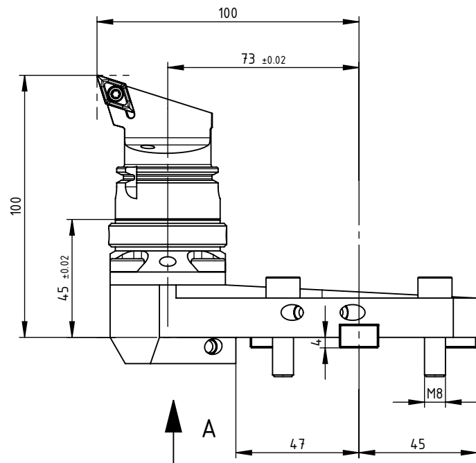
ANSICHT A
