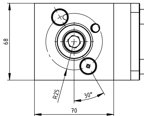
ANSICHT B (1 : 2)
