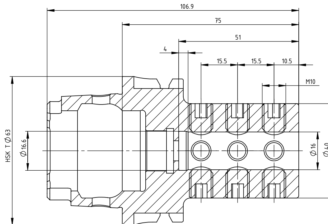
SCHNITT A-A
