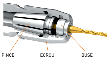
PINCE ÉCROU BUSE
